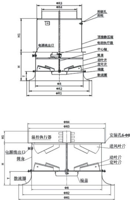
SWD630-800自动温控风口示意图
