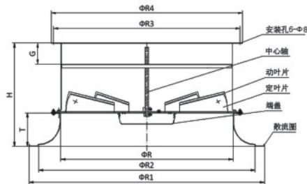
SWD200-500手动旋流风口产品示意图
