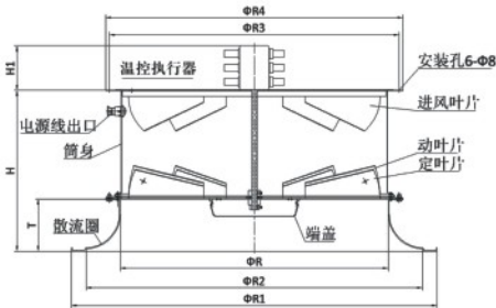
SWD630-800自动温控风口示意图
