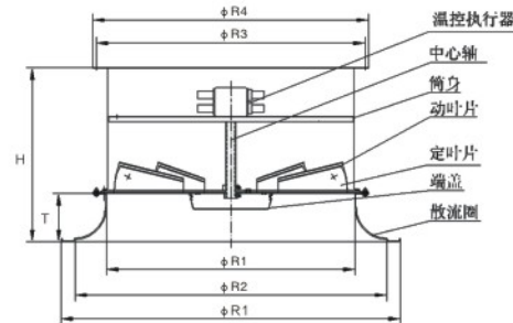
SWD200-500自动温控旋流风口示意图
