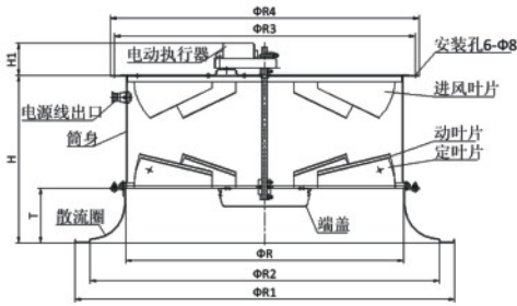
SWD 630-800电动旋流风口示意图
