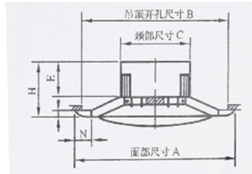
普通型安装示意图
