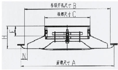
温控型安装示意图
